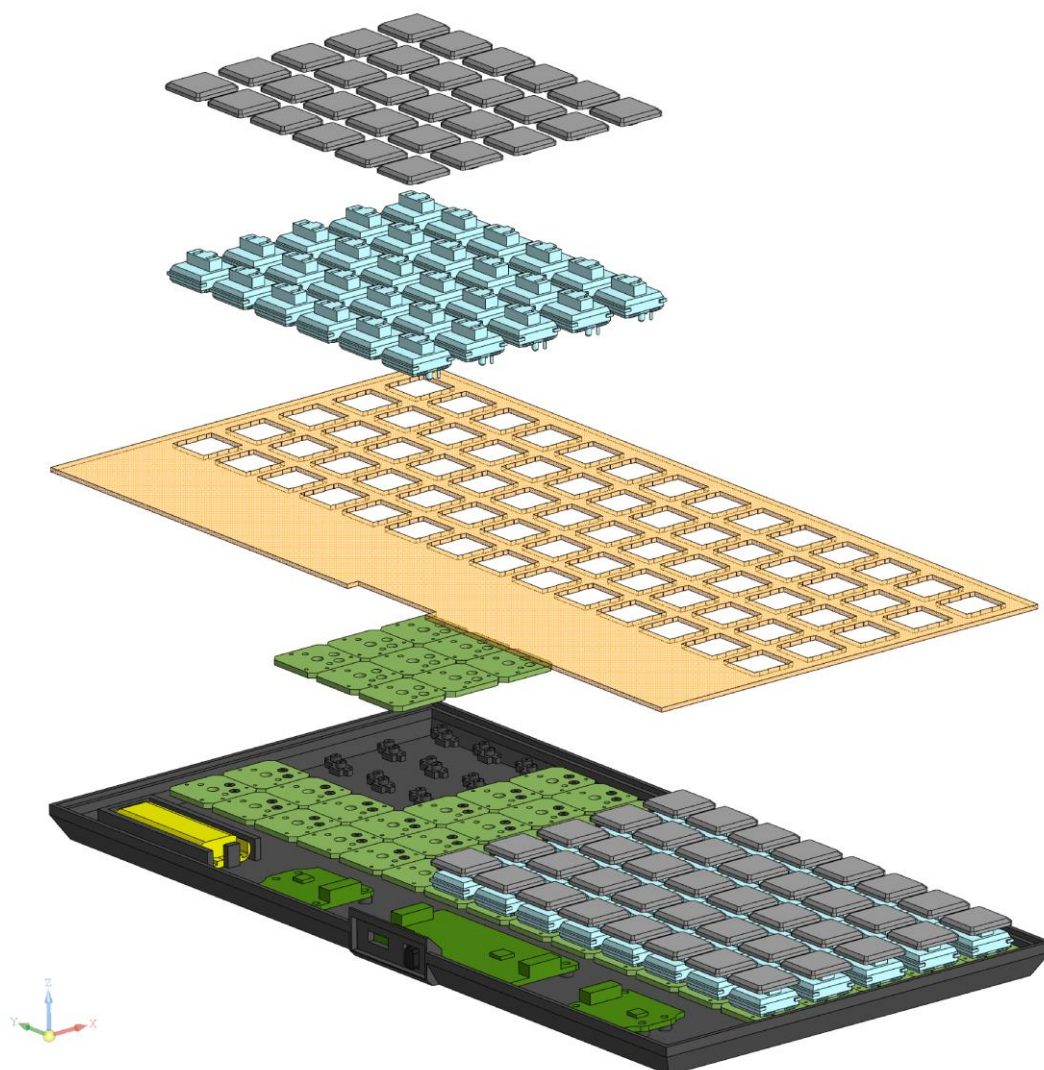
Рисунок 1 - Разнесённый вид цифровой модели клавиатуры
