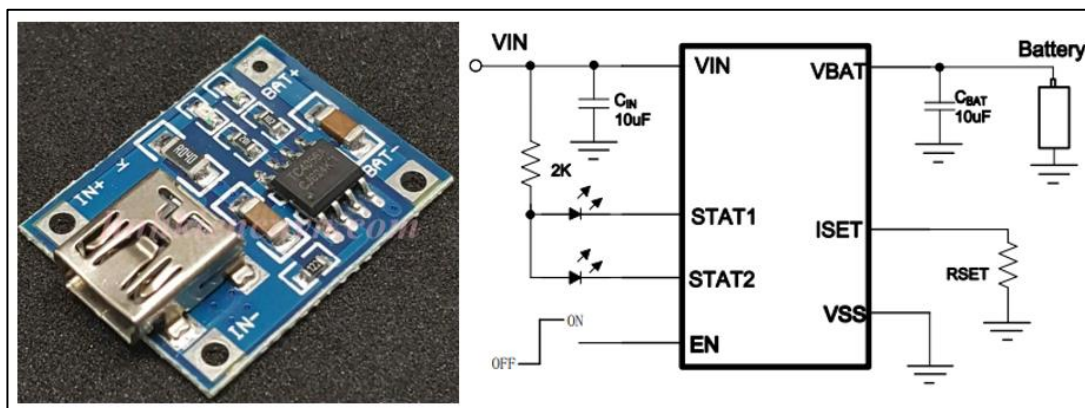
Рисунок 40 – отладочная плата TP4056 и принципиальная схема обвязки контроллера
