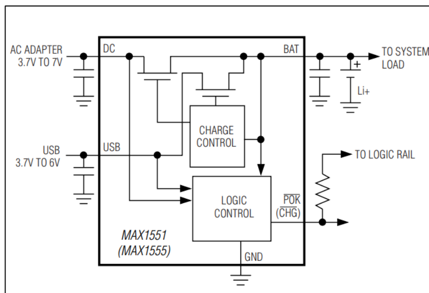
Рисунок 43 – Принципиальная схема контроллера
